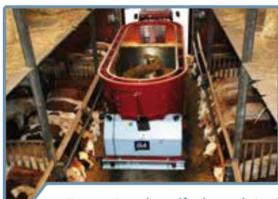
Tværgående udfodringsbånd bagpå
